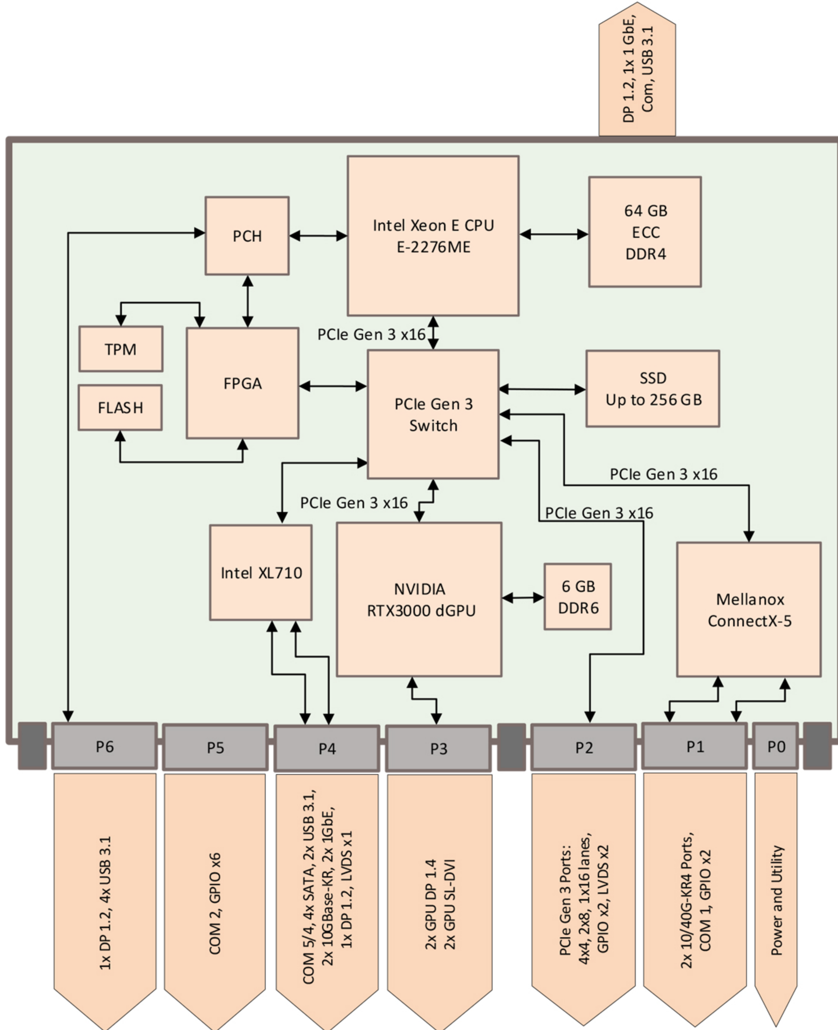
Block diagram (VITA 65)
